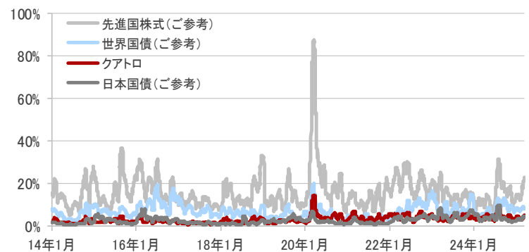
図表7:クアトロ、先進国株式、世界国債、日本国債リスク推移 日次、年率化、期間:2014年1月17日～2025年3月31日
